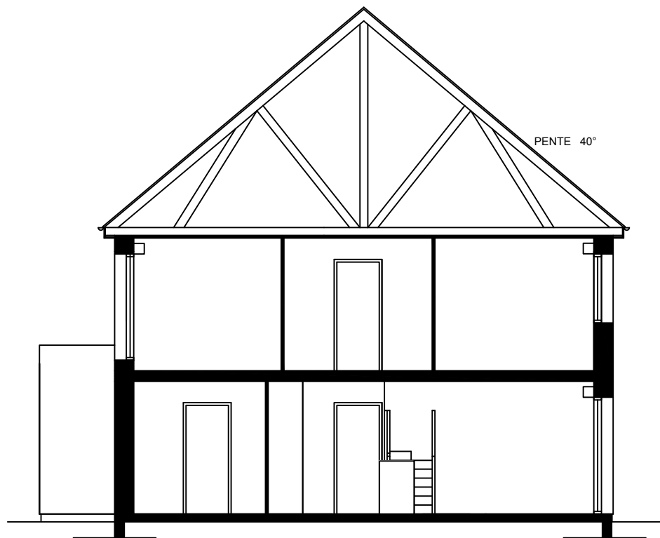
Coupe A-A
