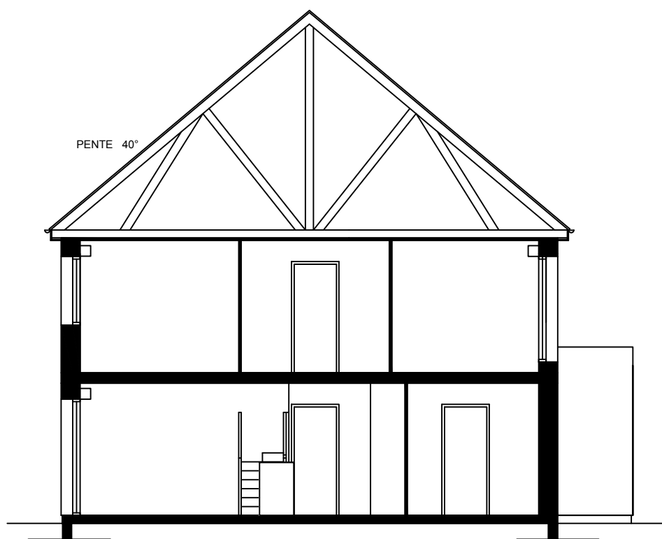
Coupe A-A
