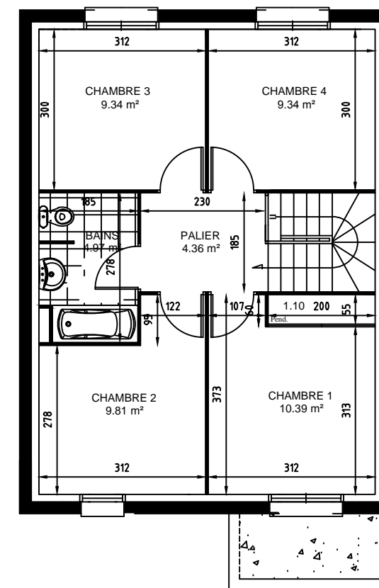
Etage
