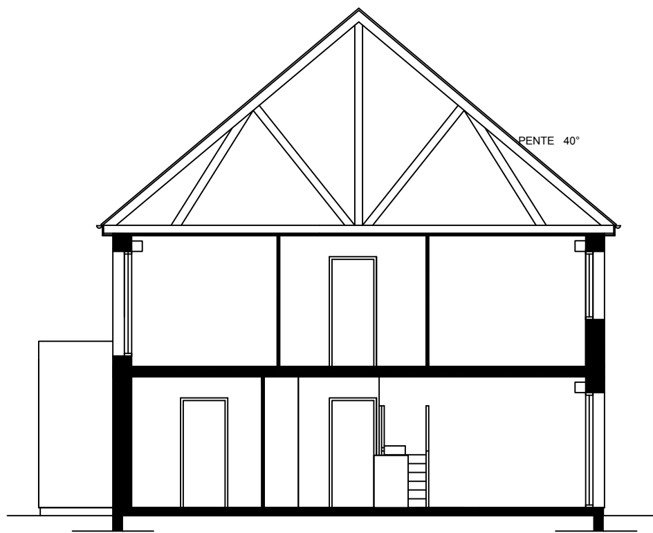
Coupe A-A
