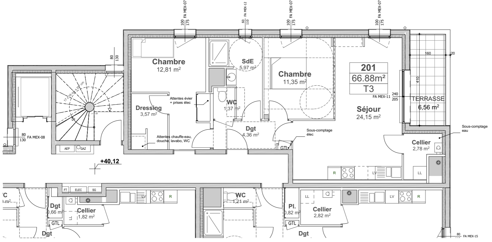
CONFIGURATION INITIALE: T3
